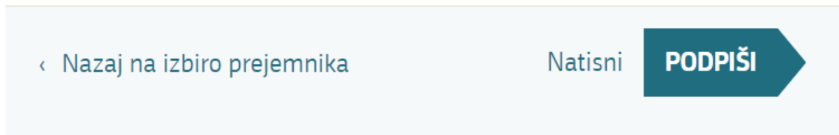
Slika 10: Podpisovanje dokumenta
